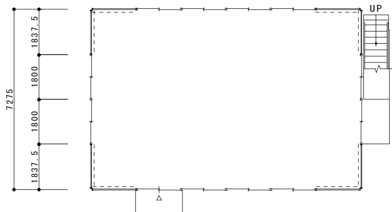
1階平面図
