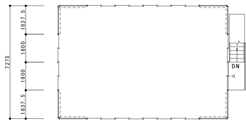
2階平面図
