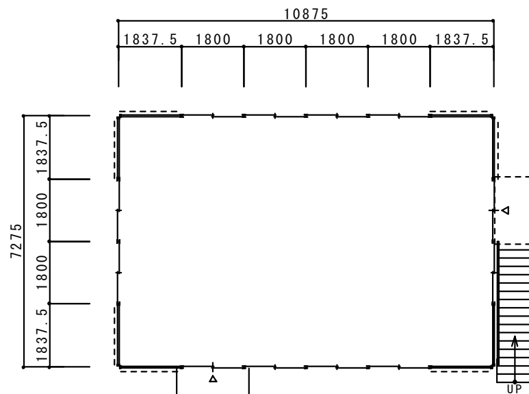
1階平面図
