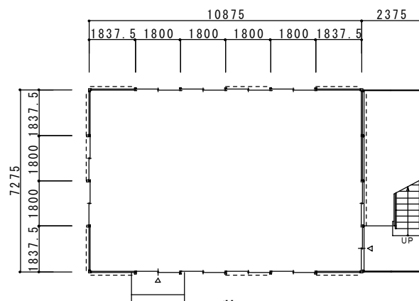
1階平面図
