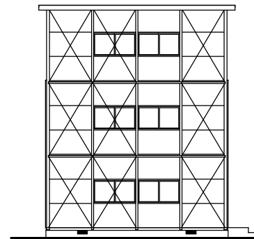
立面図
