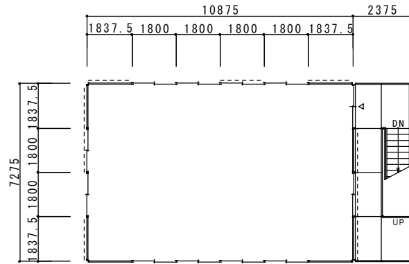
3階平面図
