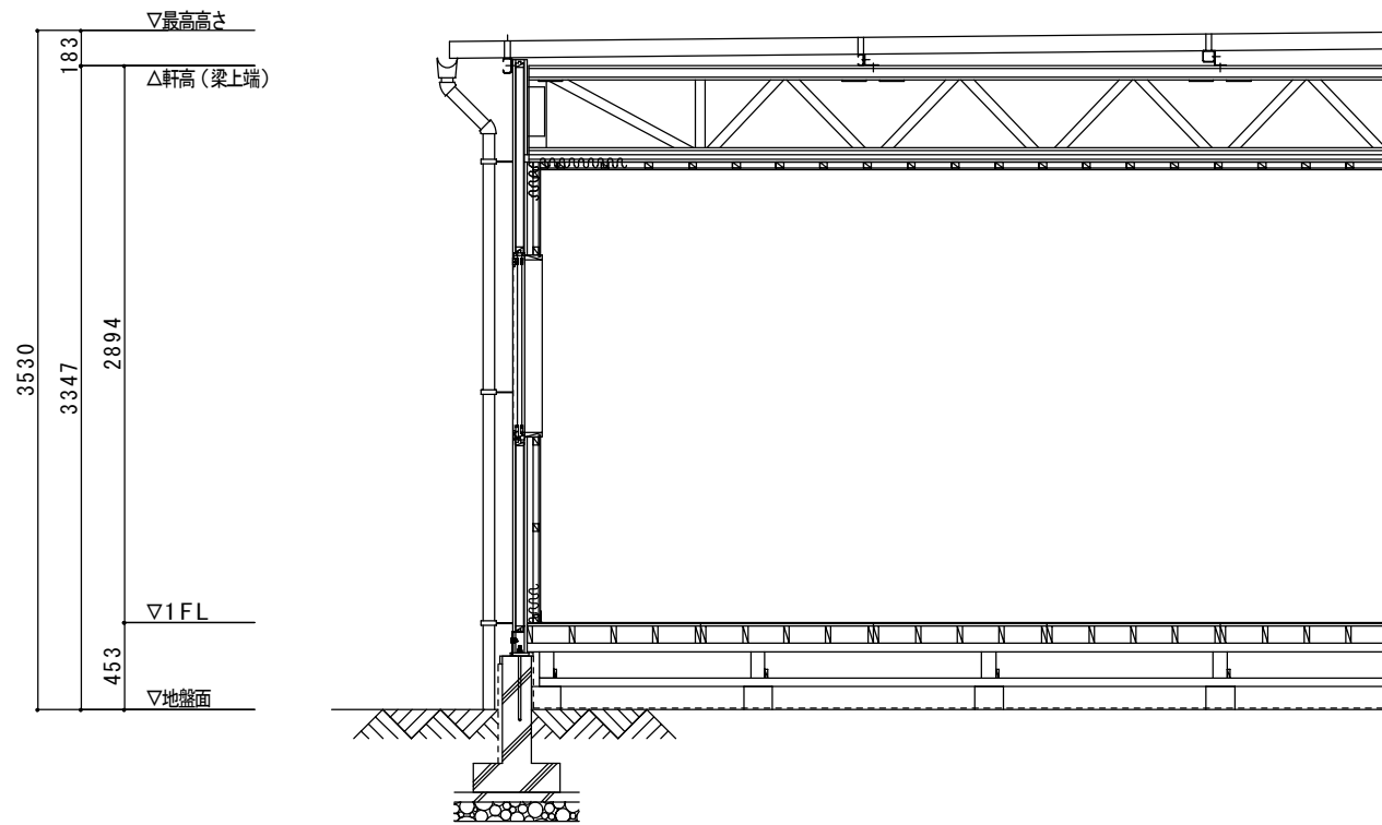
矩 計 図
