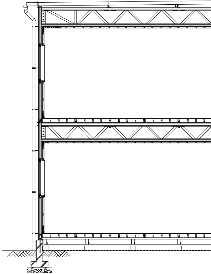
矩計図
