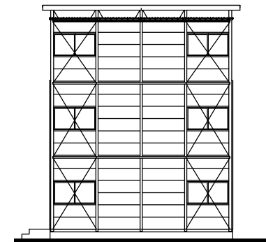
立面図
