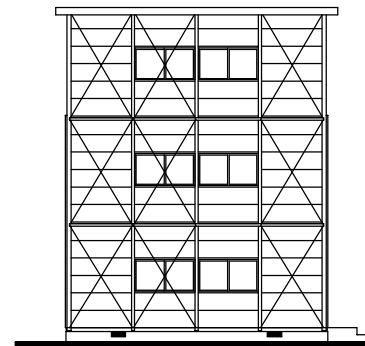
立面図
