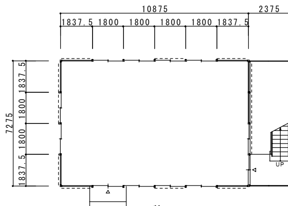
1階平面図
