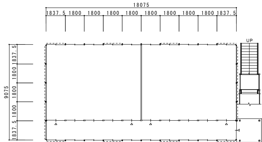
1階平面図
