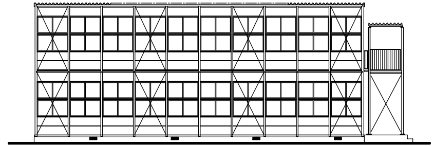
立面図
