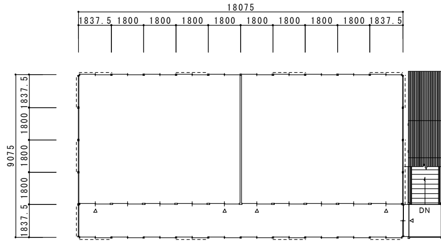
2階平面図
