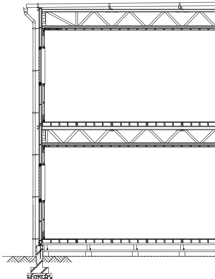
矩計図
