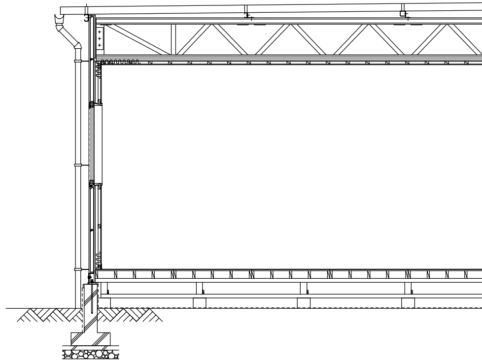
矩計図
