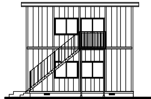
立面図
