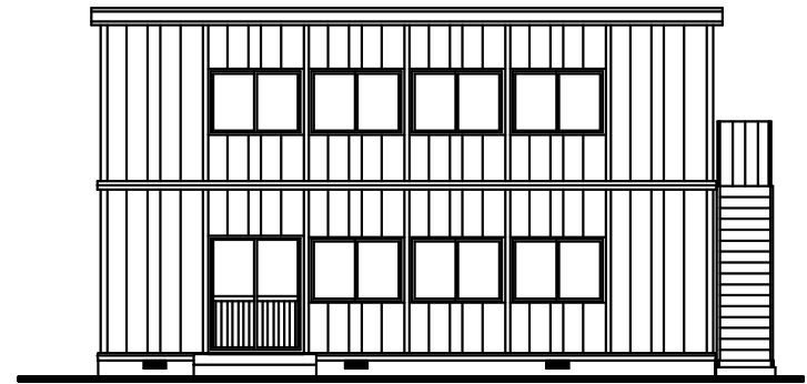
立面図
