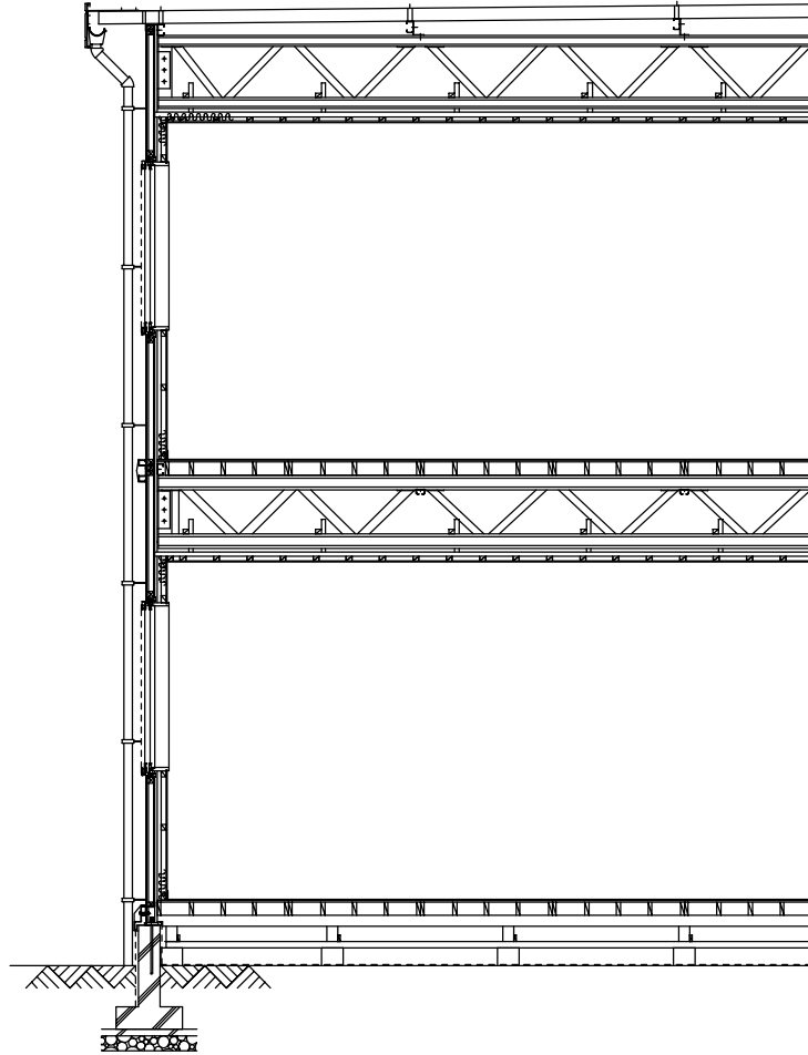
矩計図
