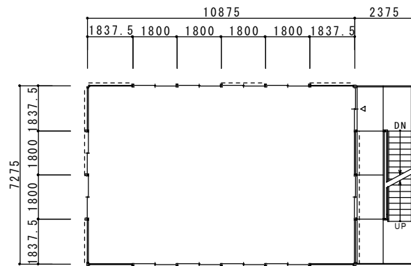
3階平面図
