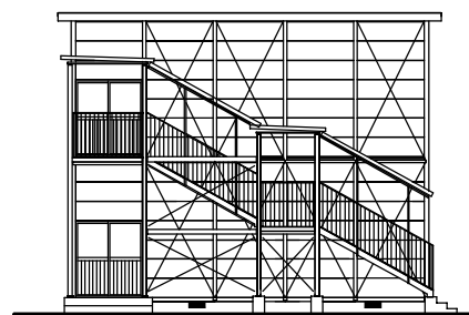
立面図
