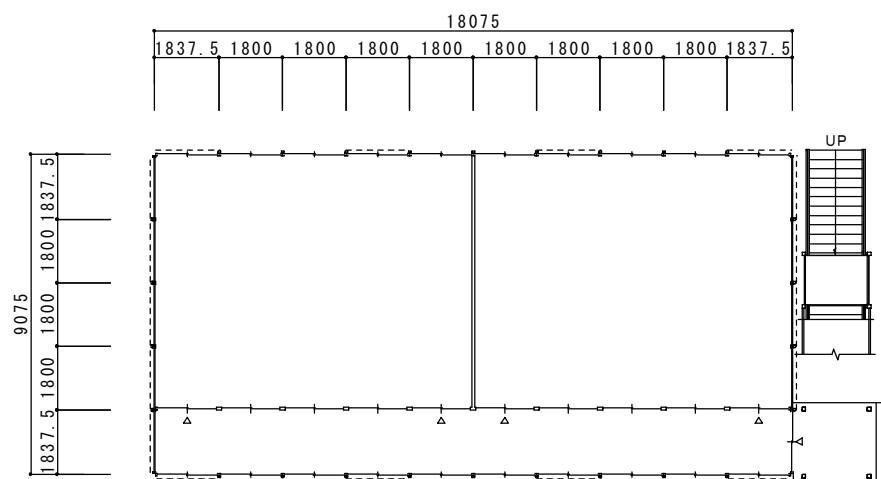
1階平面図
