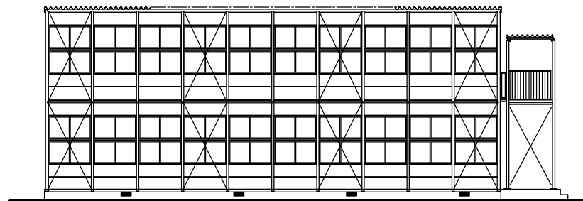
立面図
