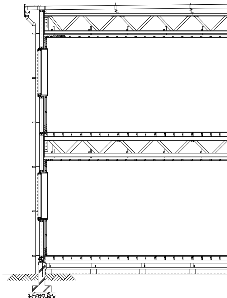
矩計図
