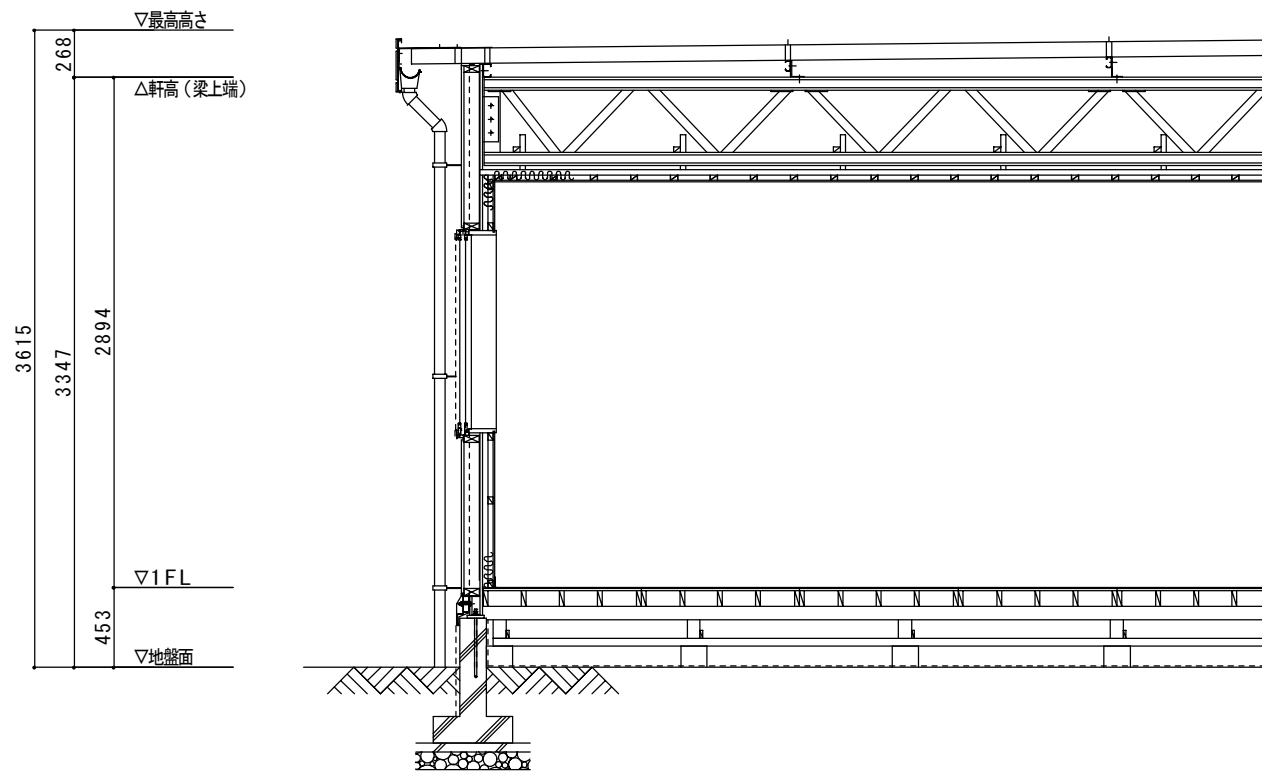
矩計図
