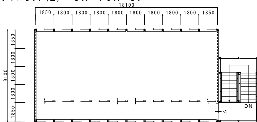
3階平面図
