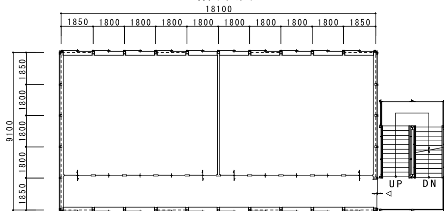
2階平面図
