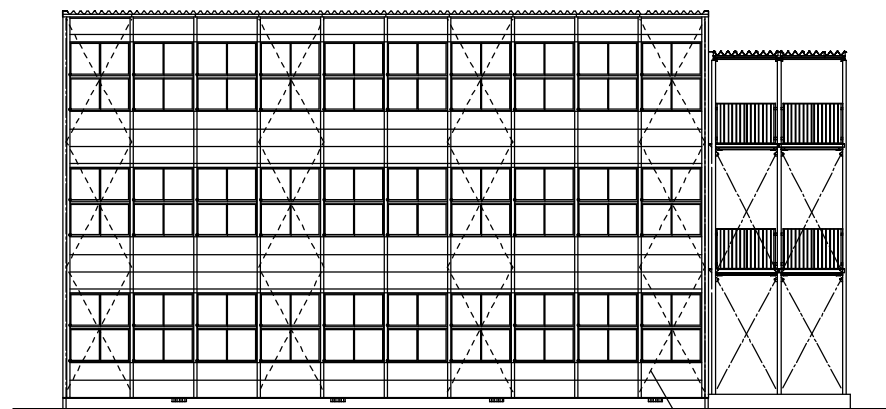
立面図
