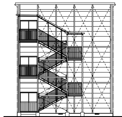
立面図
