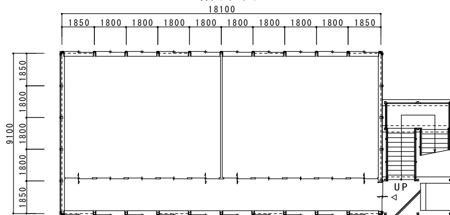
1階平面図
