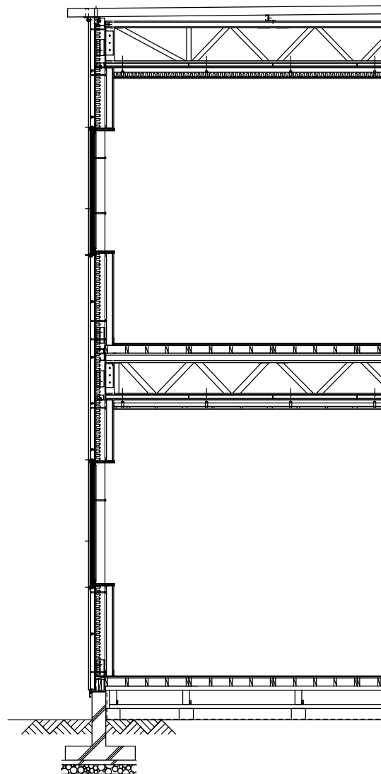
矩計図
