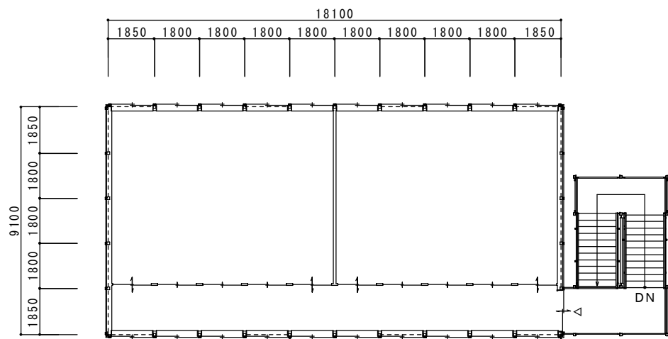
2階平面図
