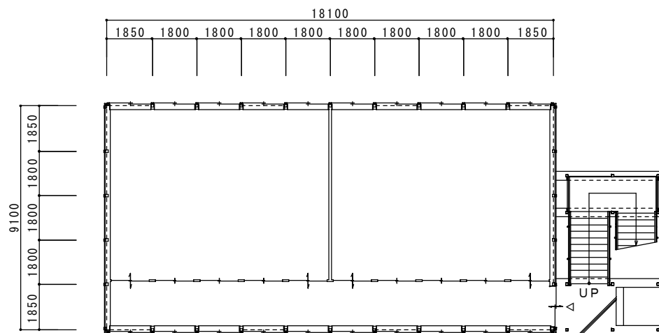
1階平面図
