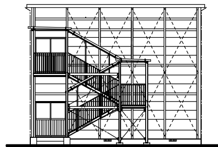
立面図
