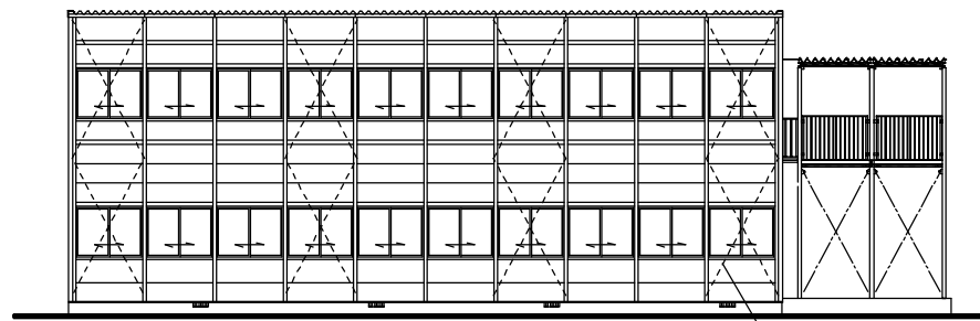
立面図
