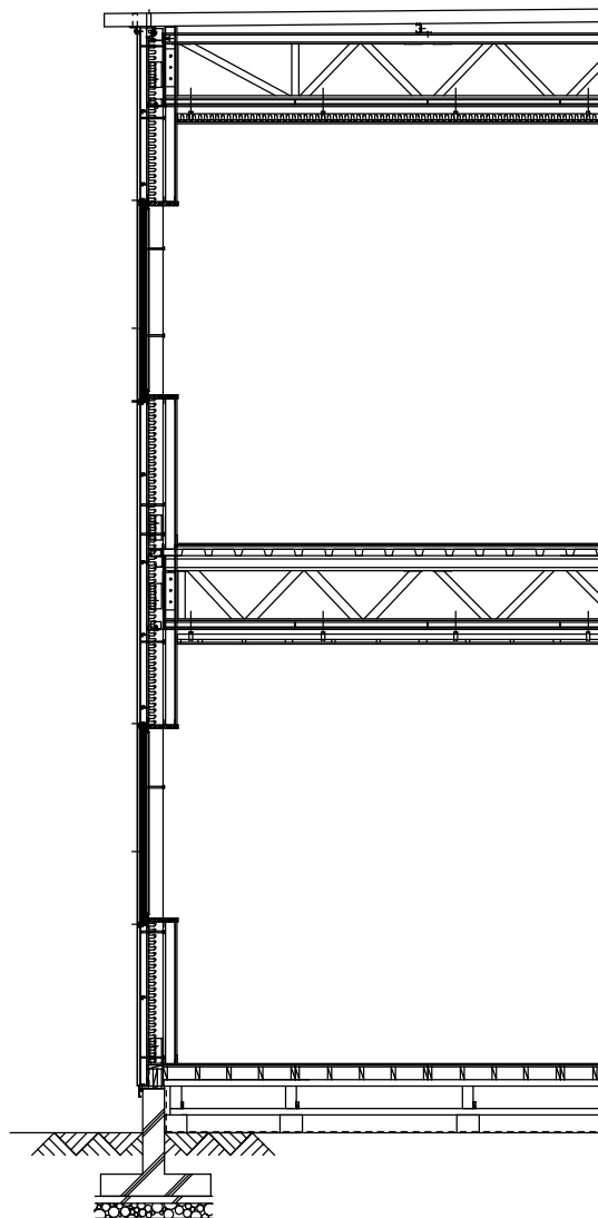
矩計図
