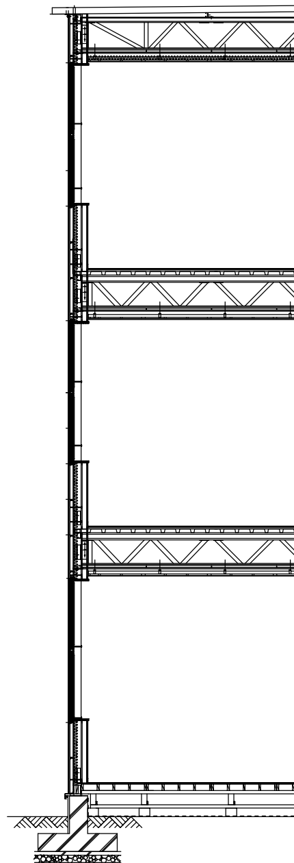
矩計図
