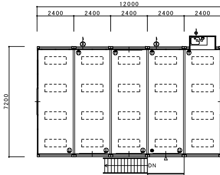
2階平面図
