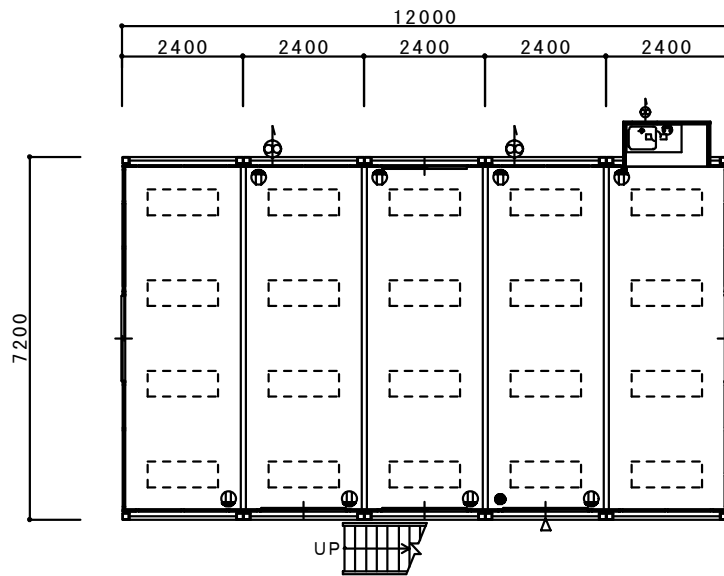
1階平面図
