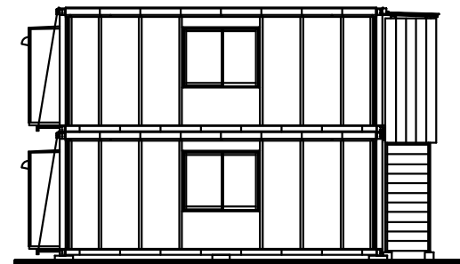
立面図
