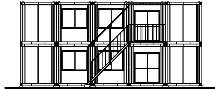
立面図
