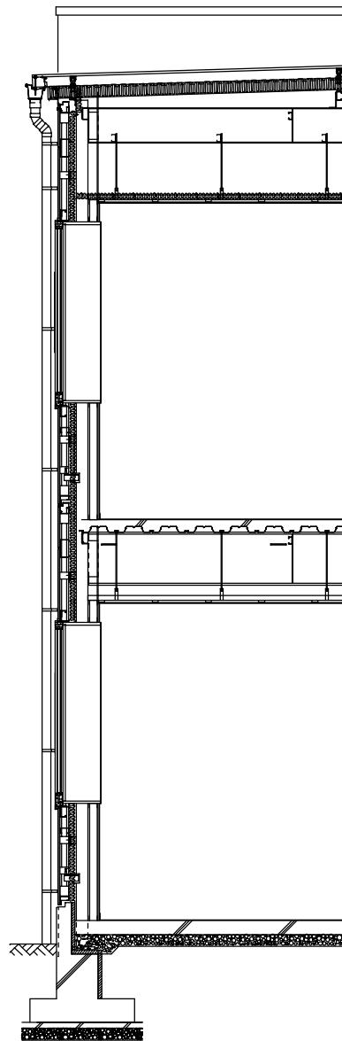
矩計図
