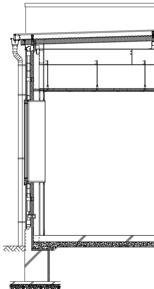
矩計図
