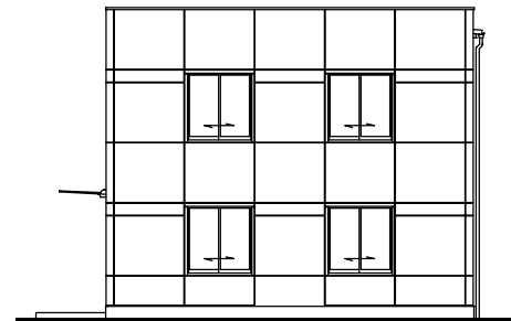
立面図
