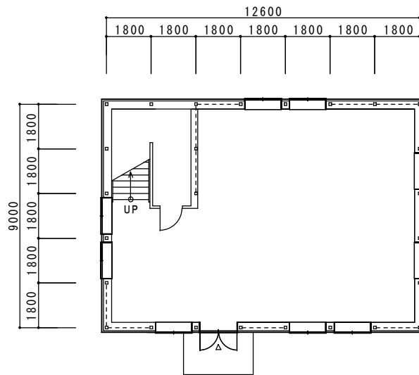
1階平面図
