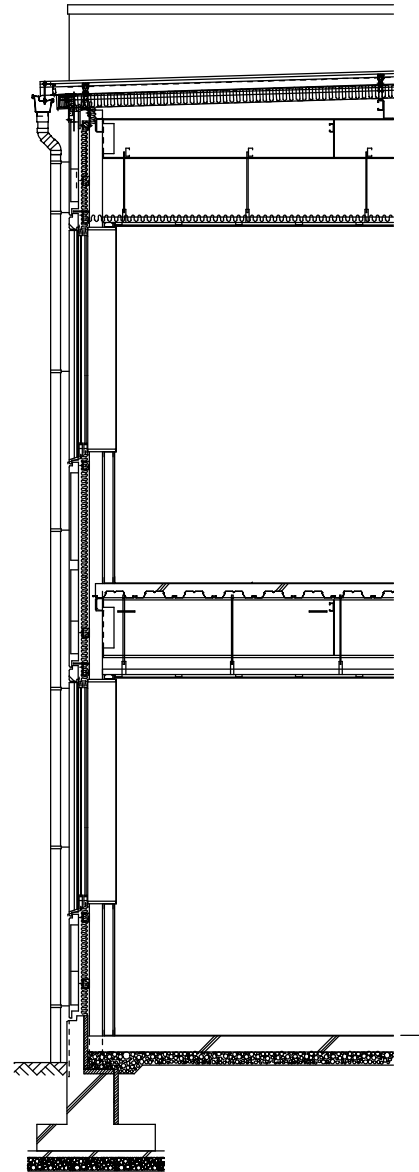
矩 計 図
