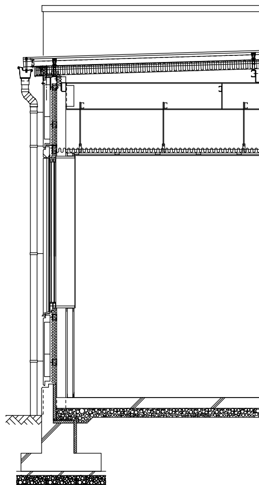
矩計図
