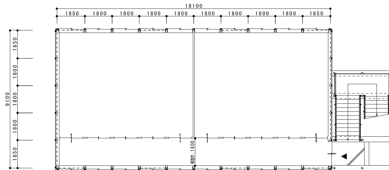
1階平面図
