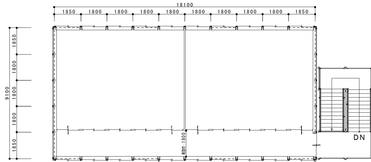
3階平面図
