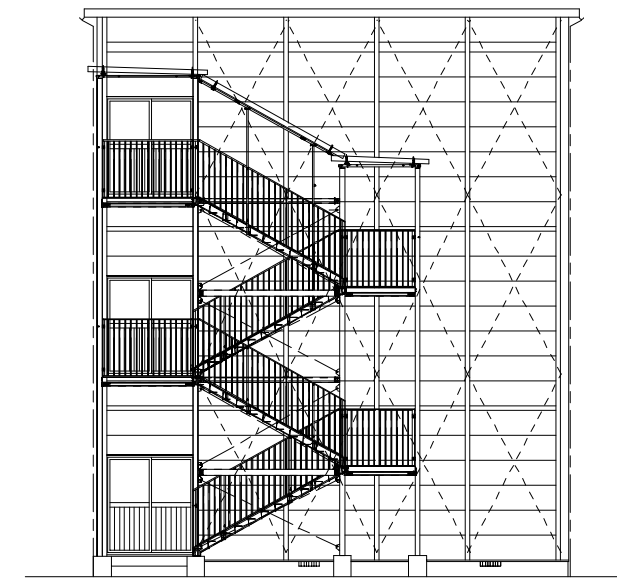
立面図
