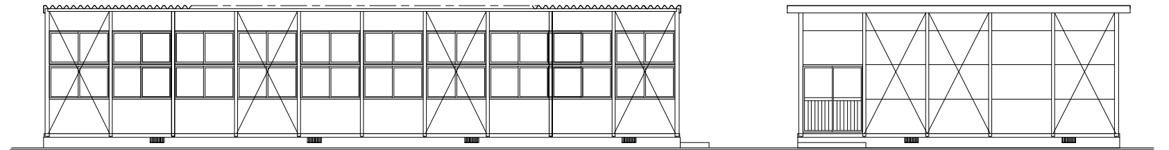
フラットスタンダード(L) 立面図
